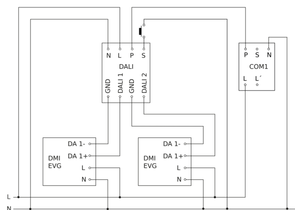
Schéma du circuit d'interconnexion maître/esclave
